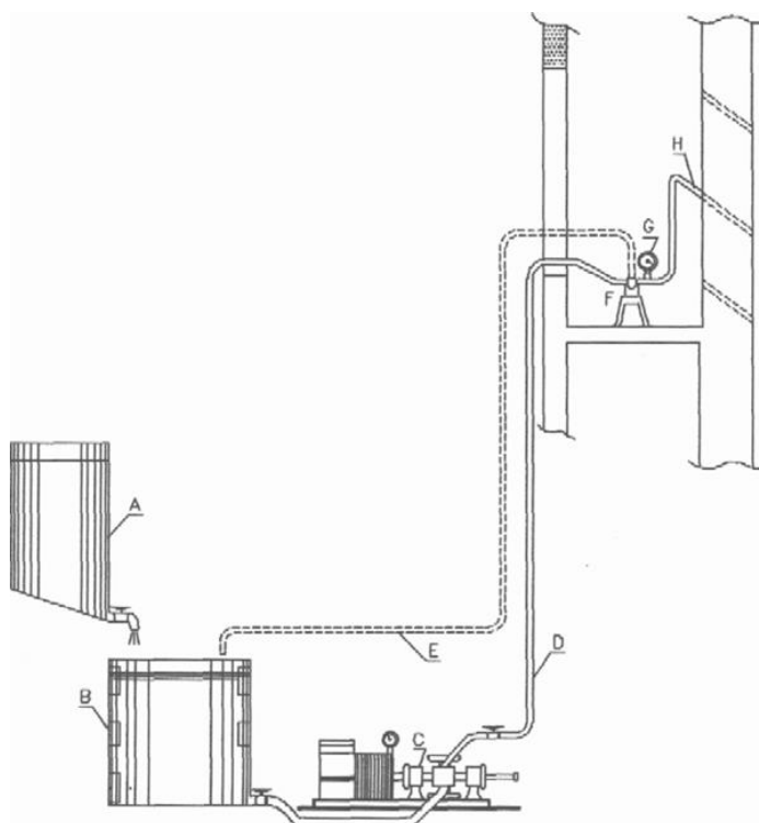
Σχηματική απεικόνιση εξοπλισμού προετοιμασίας και εισπίεσης ενεμάτων
